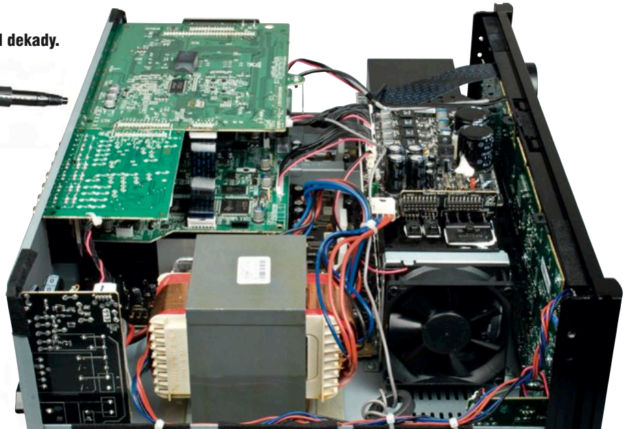
Radiator tunelowy z wentylatorem.
